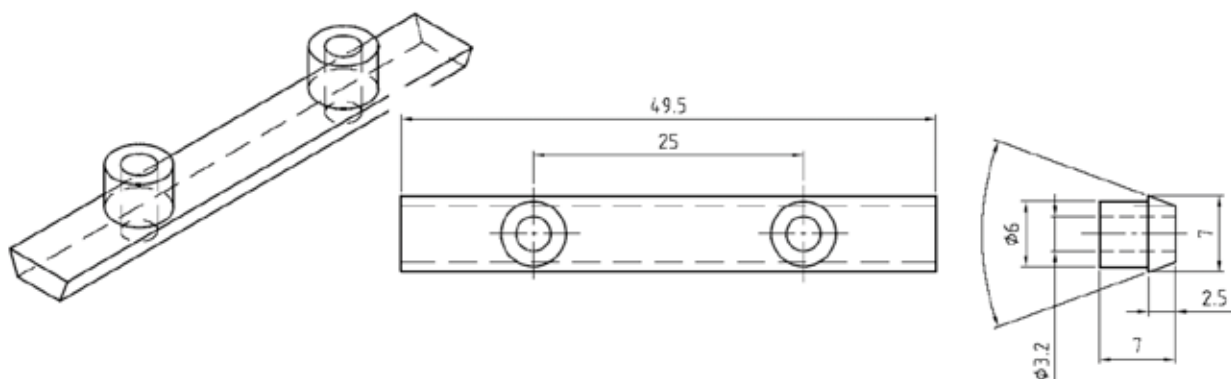
Indlægsskinne af polyamid eller messing M4 L=50 mm
