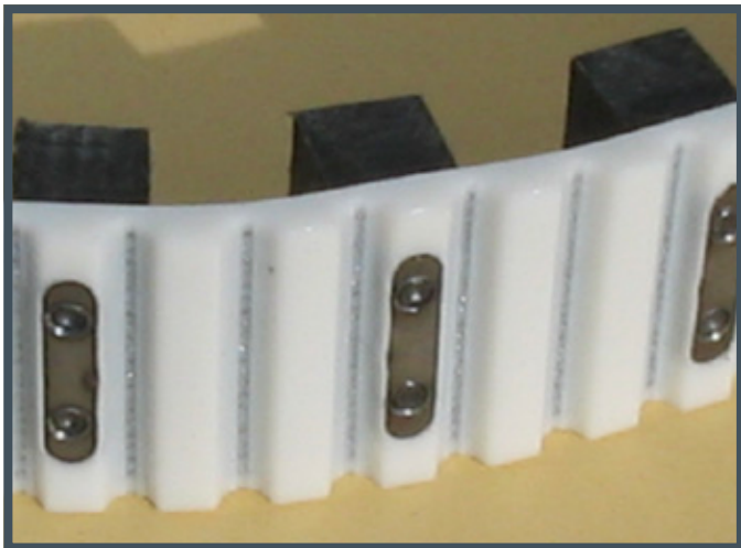
Set fra tandsiden
